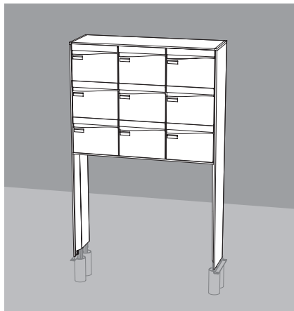
b Doppelstütze zum Einbetonieren
